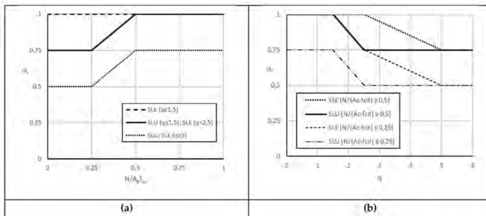
Figura C7.2.5 Dipendenza di \alpha_s dal carico assiale N e dal fattore di comportamento q .
